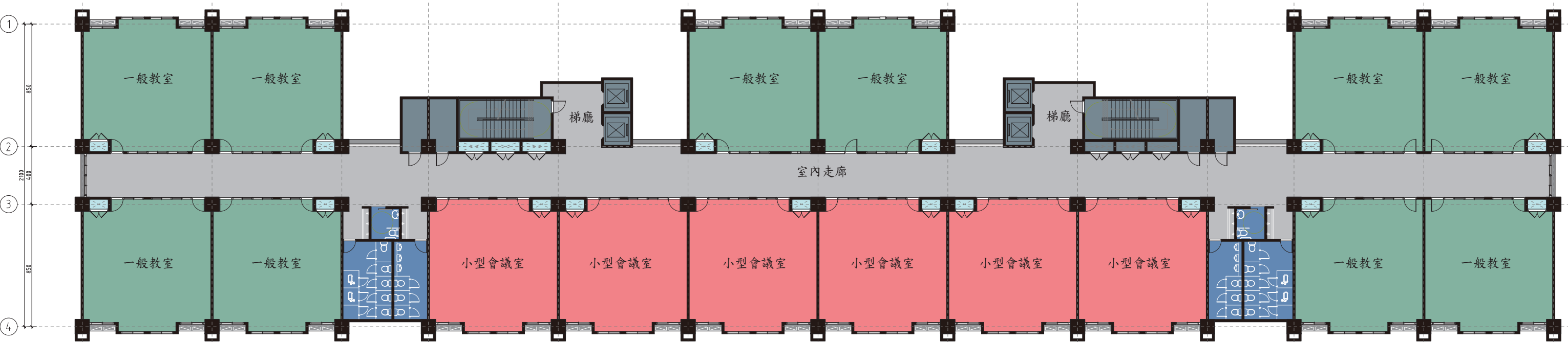
二層建築平面配置圖 A3=S：1/300
