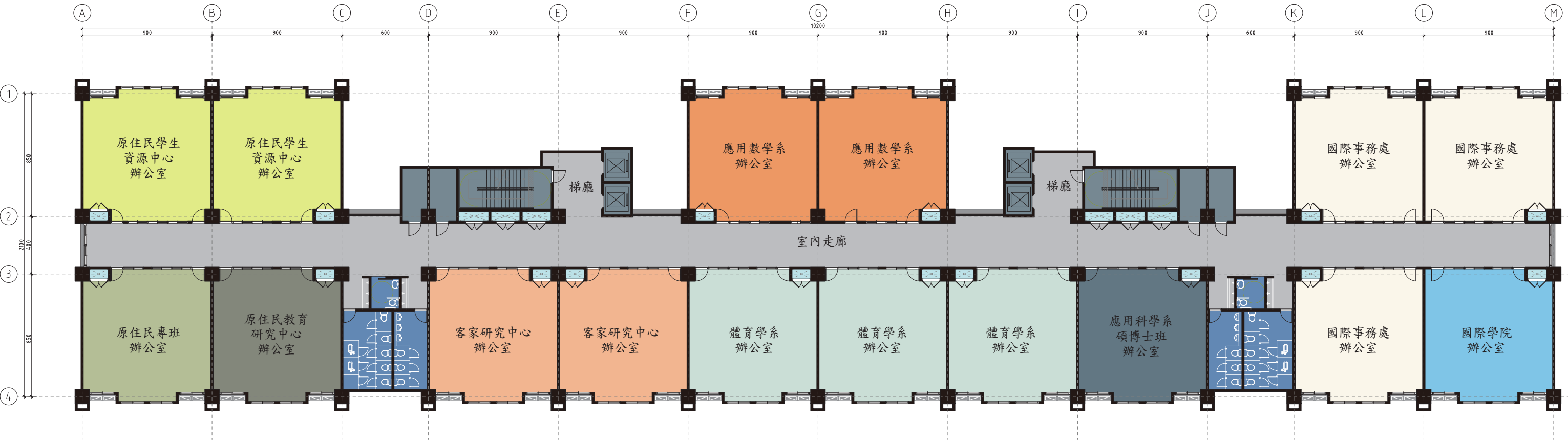
六層建築平面配置圖 A3=S：1/300
